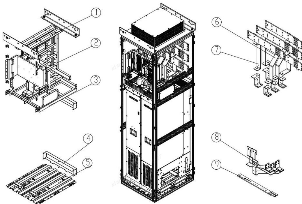
图 4-11 整流回馈柜结构布局图
