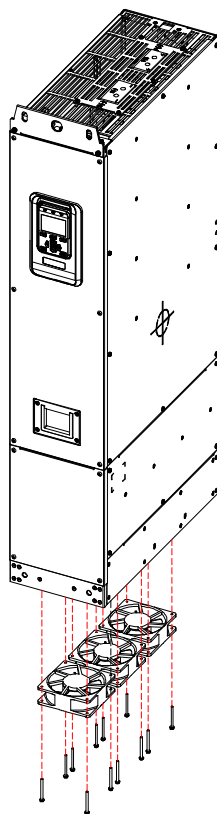
图 5-3 B4/B5 机型风机更换图
