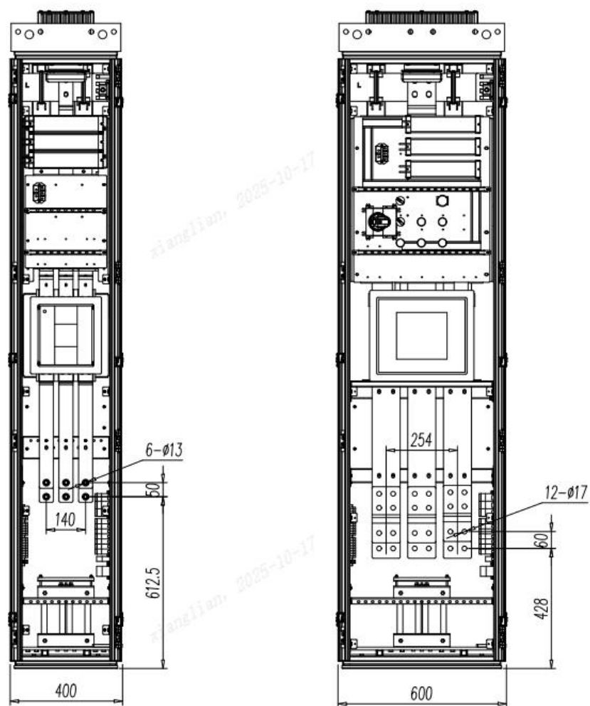
图 4-4 进线柜尺寸 (单位: mm)
