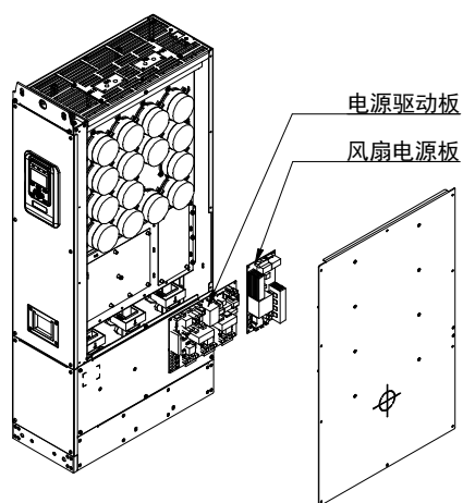
图 5-9 B4 机型电源驱动板及风扇电源板更换图
