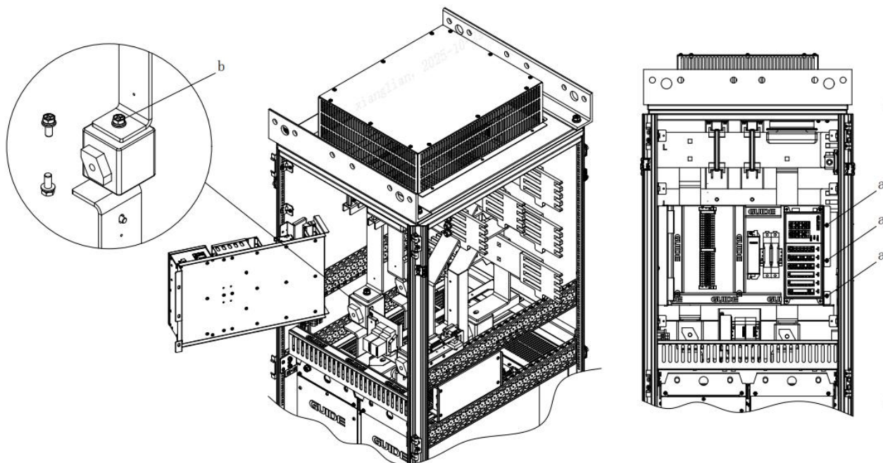
图 5- 2 熔断器更换
