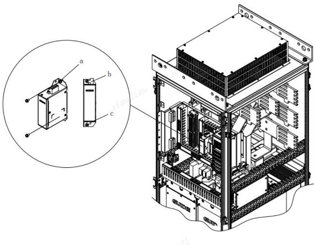
图 5-1 电源采样模块更换
