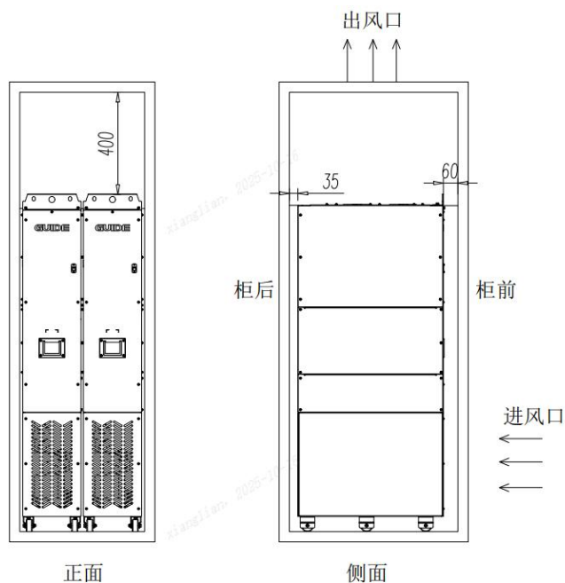
图 2- 4 风道要求（单位： mm）
