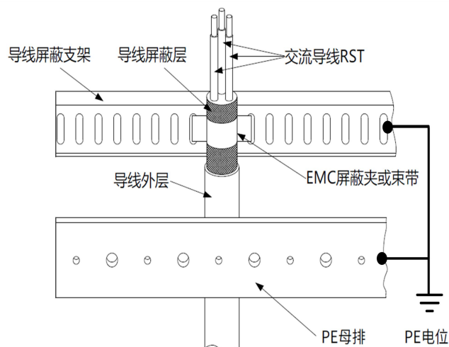
图 2-6 屏蔽型功率电缆连接要求示意图
