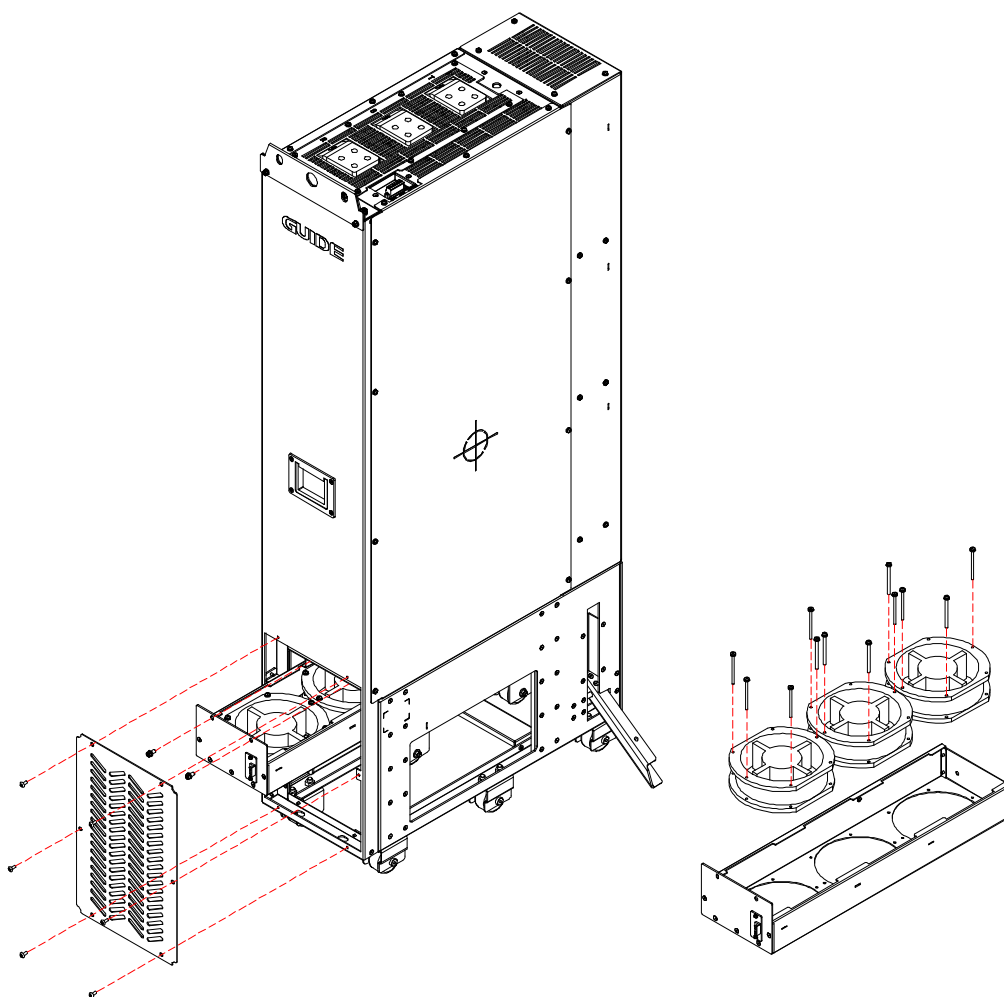
图 5-6 LCL 滤波模块风机更换图
