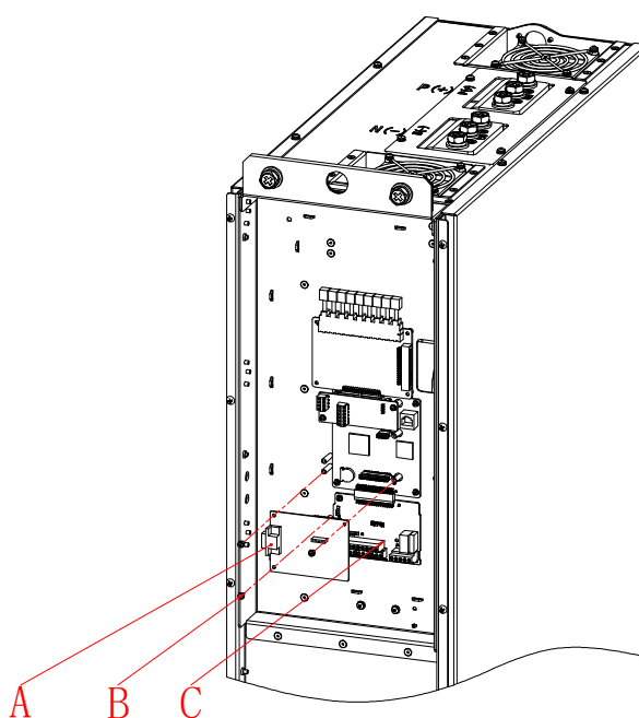
变频器 DP 的安装与接地
