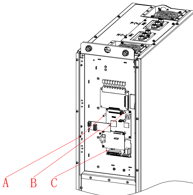
变频器 PG 卡的安装与接地
