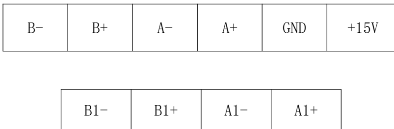
接线端子示意
