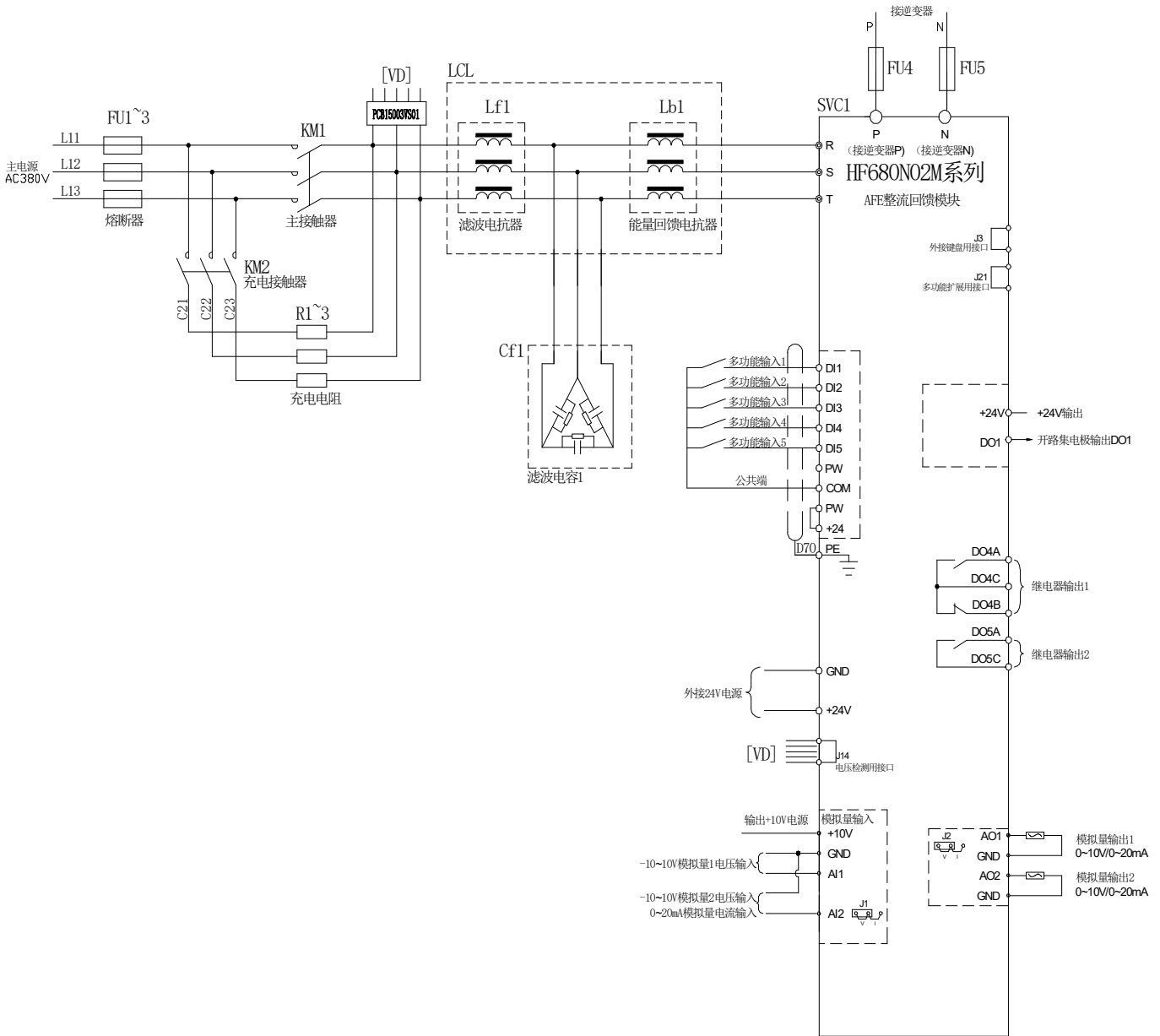
整流回馈单元的单机主回路图：
